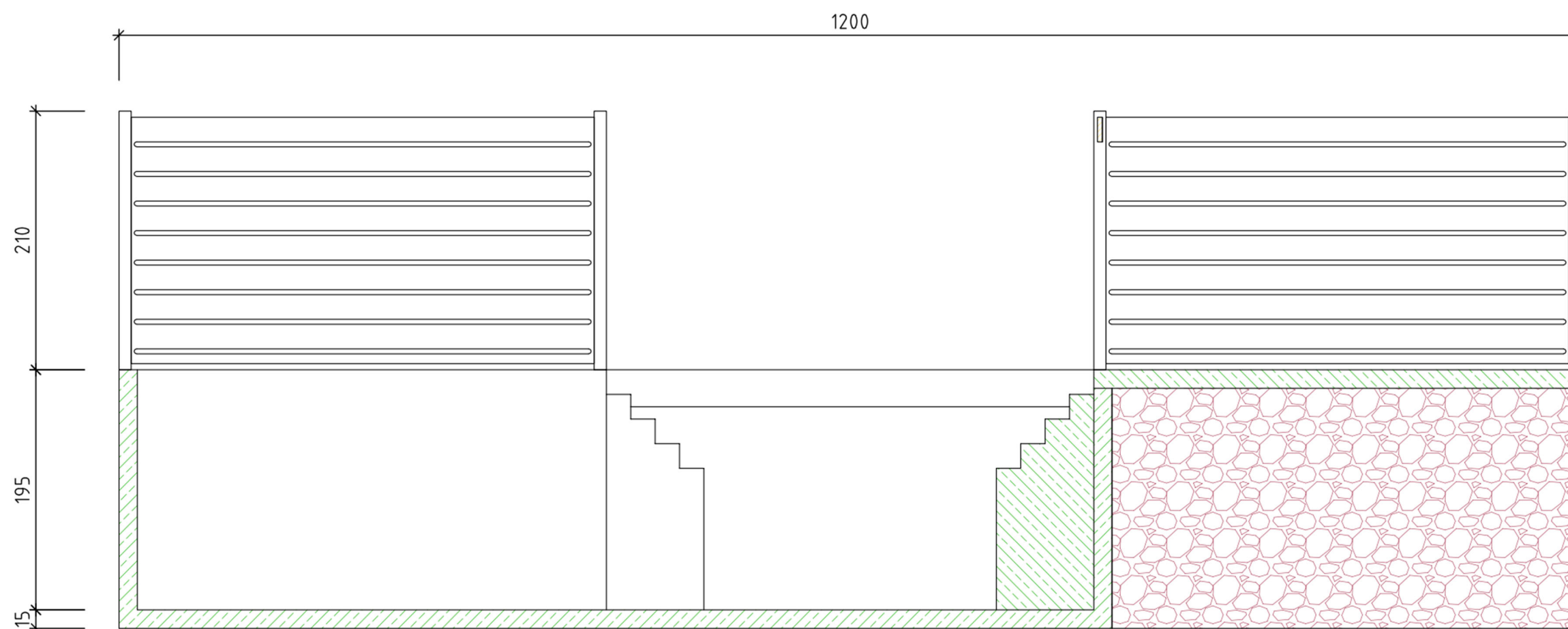
Schnitt_A-A
