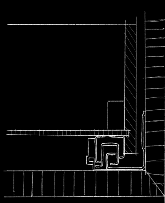
LADE - AUFRISS
